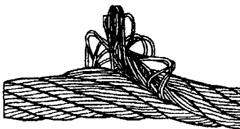
Рисунок 11. Выдавливание сердечника
